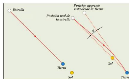
Desplazamiento de Einstein
